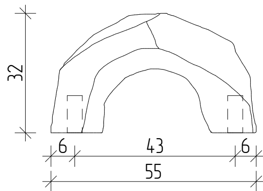
Вид сбоку
