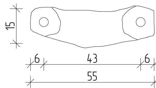
Вид снизу
