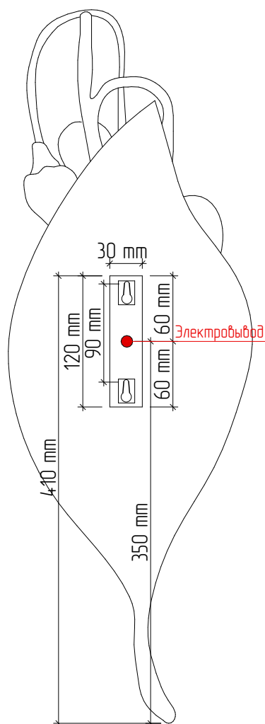
Вид сзади
